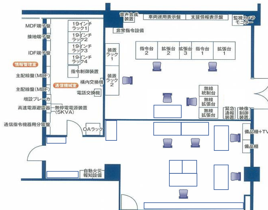
西胆振行政事務組合消防本部 2階通信機械室/通信指令室レイアウト
